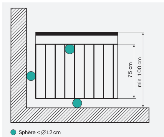
Illustration 9 Garde-corps à barreaux verticaux
